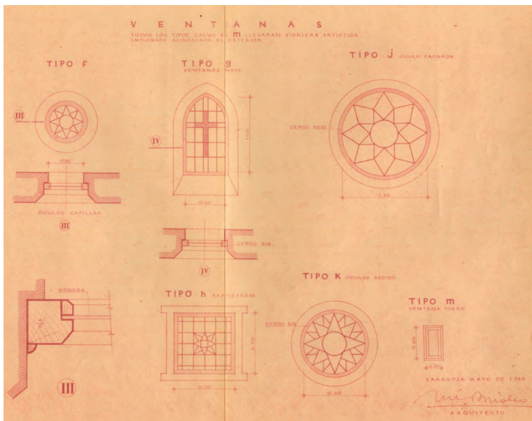
5. José Borobio. Diseño de vidrieras para la iglesia de El Temple, mayo de 1948. Fuente AHPProvZ.
