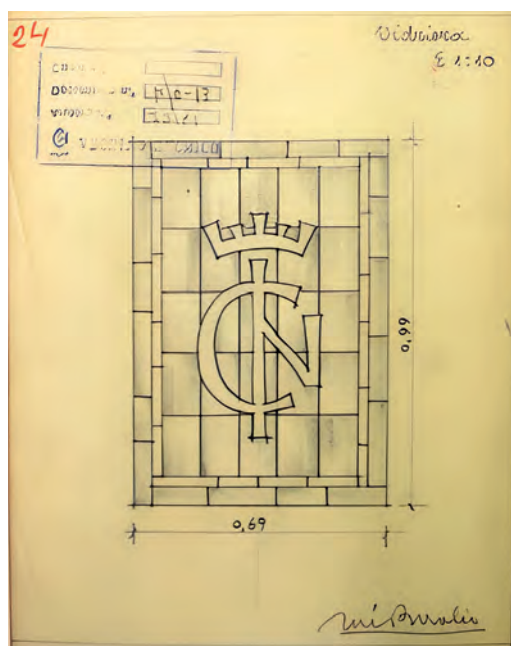
2. José Borobio. Diseño de vidriera para la residencia del INC en la finca Paridera Alta y Baja, 1946. Fuente AHPProvZ.
